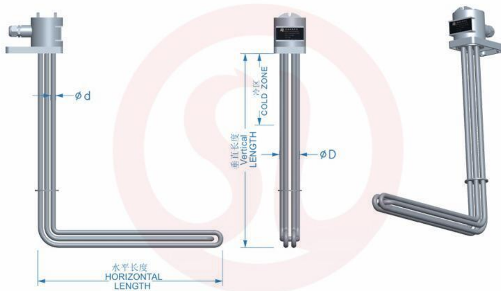
L型三管组合式铁氟龙液体加热器
